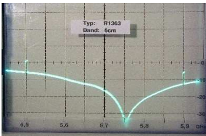
SWR 6cm
