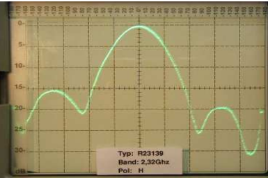
Öffnungswinkel H13cm
