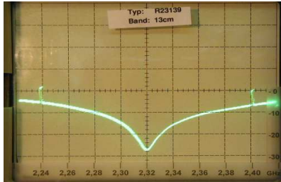
SWR 13cm
