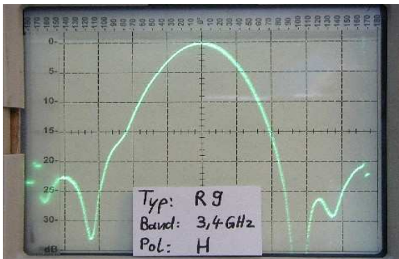
Öffnungswinkel H
