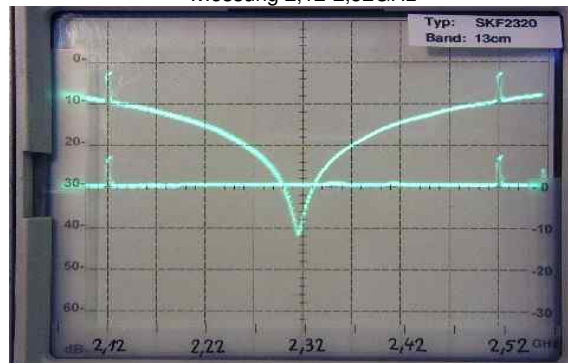
Messung 2,12-2,52GHz
