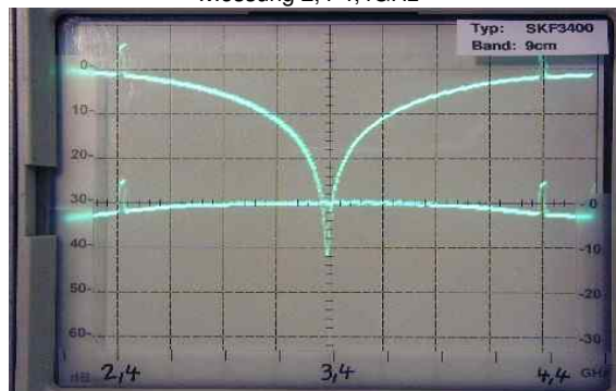
Messung 2,4-4,4GHz
