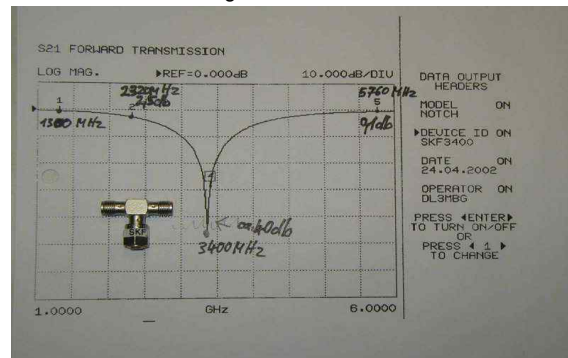
Messung 1-6GHz
